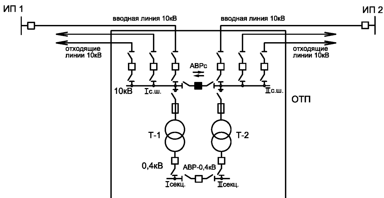
Рисунок 2 - Схема присоединения ТП 10/0,4 кВ, питающей потребителей категории 1
