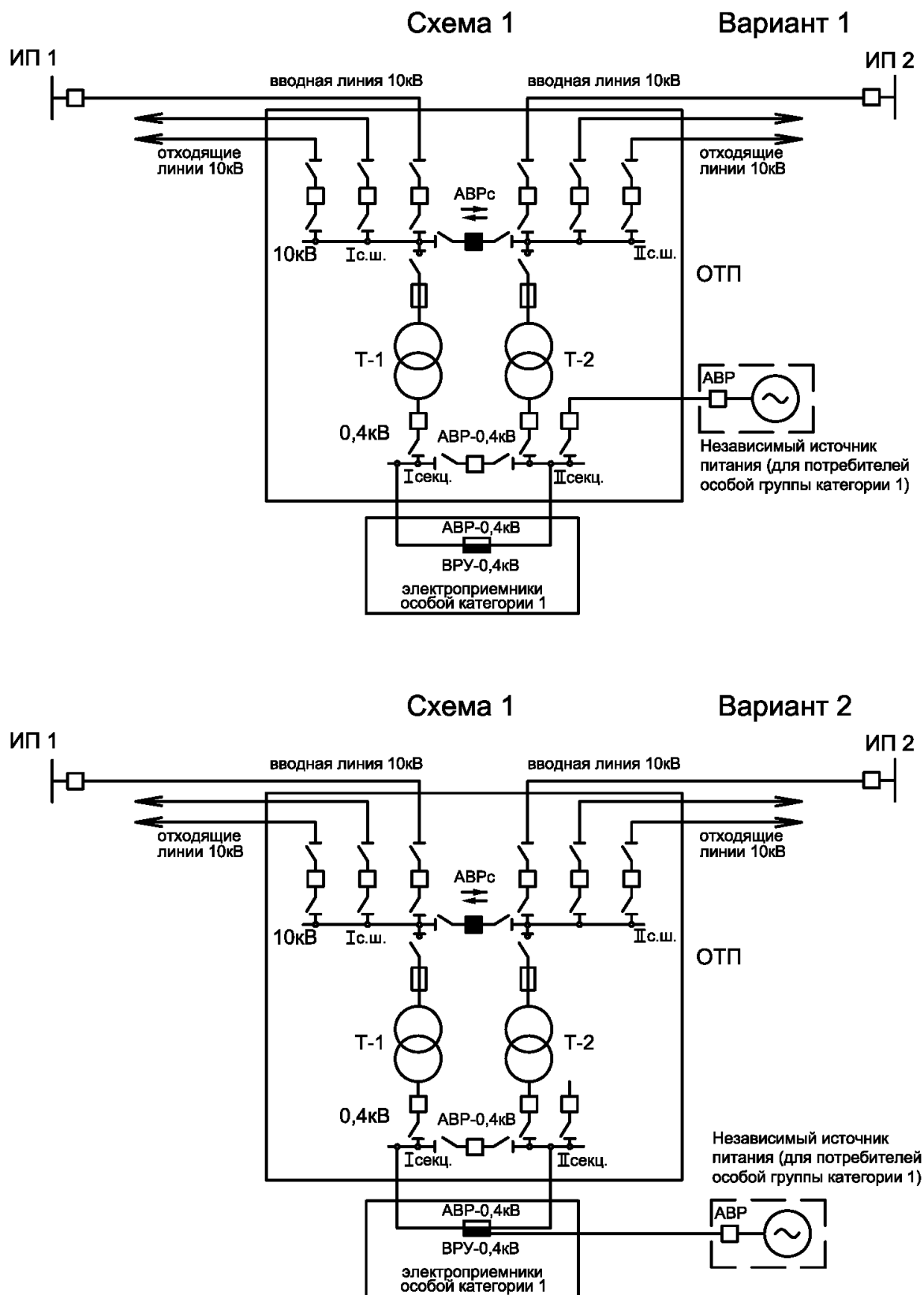
Рисунок 1 - Схемы вариантов присоединения ОТП 10/0,4 кВ, питающей потребителей особой группы категории 1
